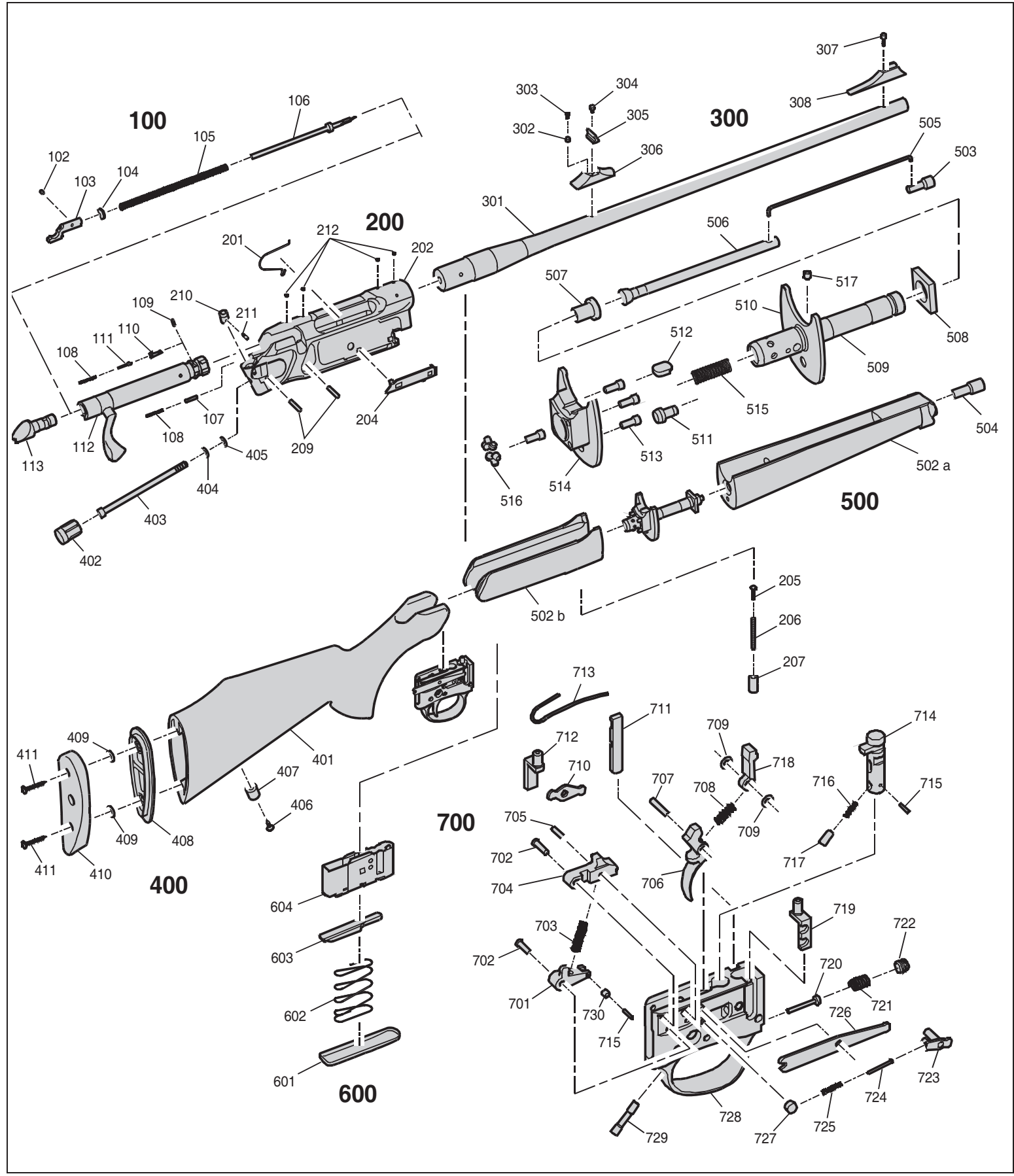
Fig. 25, Reservdelar för Sauer 202 Take Down
